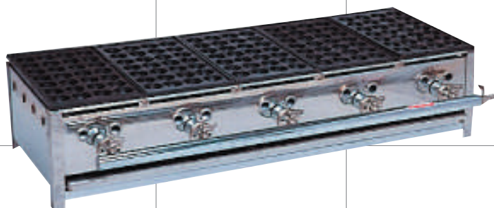
■小型たこ焼き機 84個 W560×D350×H230mm
