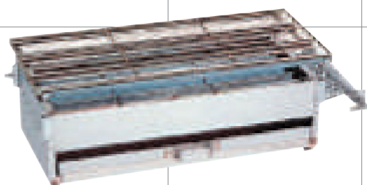
■焼き鳥機 5本バーナー W600×D270×H170mm
